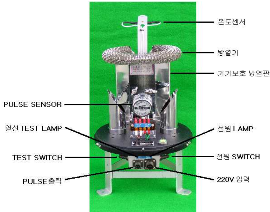
그림.1 강우설량계 내부
